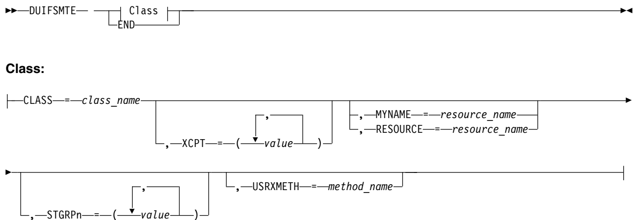
Figure 26. Macro DUIFSMTE Syntax
